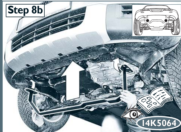
with plastic acoustic protection / mit Schallschutz Kunststoff / avec une protection acoustique en plastique
