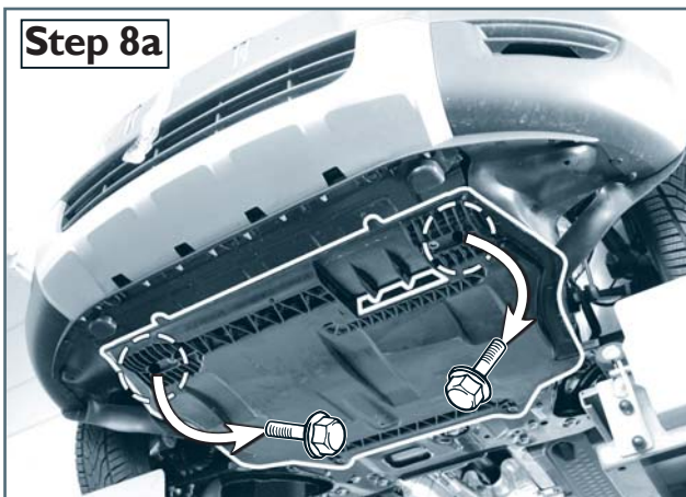
with plastic engine guard plate / mit Triebwerk- schutz Kunststoff / moteur avec protection en plastique
